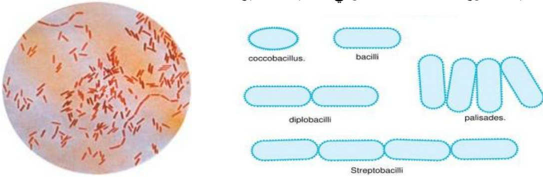
الشكل (3-5) أشكال العصيات وجراثيم Salmonella typhi التي تسبب مرض التيفوئيد
