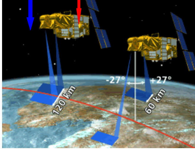
مشهد المستشعر HRV
