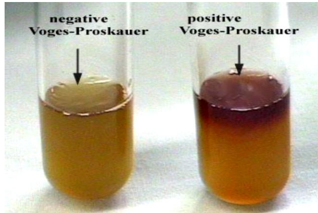
الشكل (2-8): اختبار فوكس-بروسكاوير
