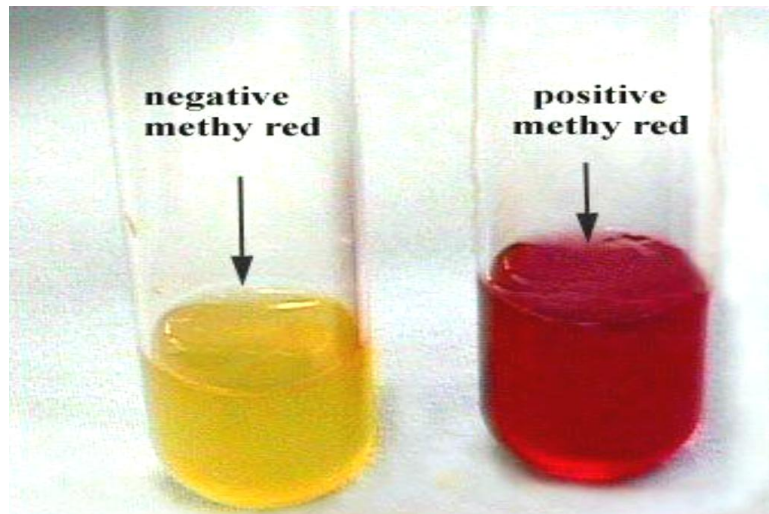
الشكل (3-8): اختبار أحمر الميثيل
