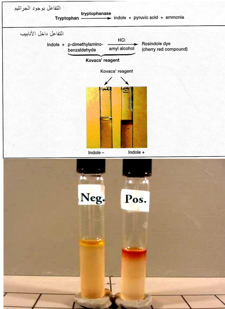
الشكل (4-8): اختبار إنتاج الإندول
