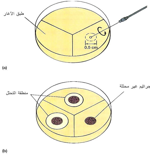
الشكل (8-6): وجود حالات شفافة حول الجراثيم المحللة للكالزئين (a) تلقيح الطبقة بالجراثيم المراد اختبارها، (b) ظهور حالات شفافة تعني حلمهة الكالزئين
