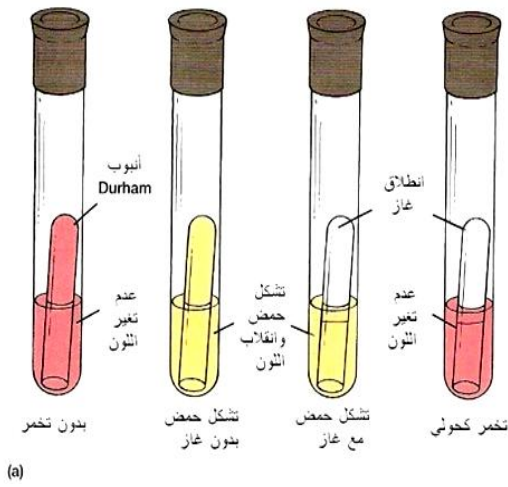
الشكل (1-8) اختمار السكريات
